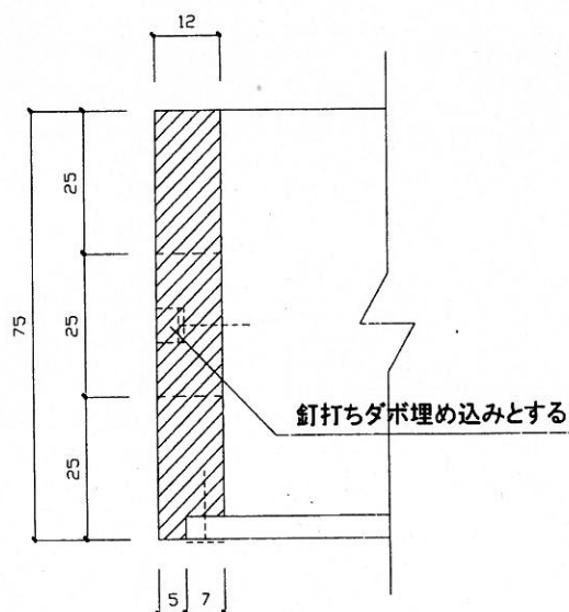
D-D' 断面図 S=1/1
