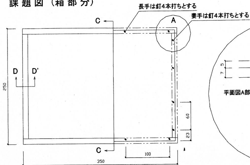
平面図 S=1/3
