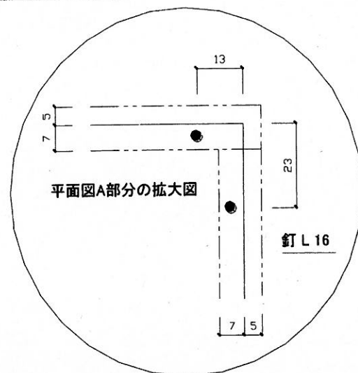
底板取付図 S=1/1
