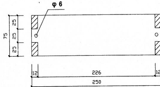
妻手側面図 S=1/3
